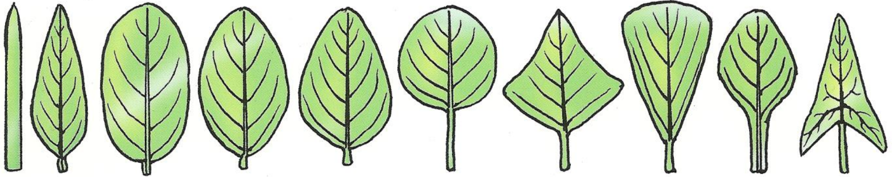
Linear 線形 Lanceolate 披針形 Oblong 長圓形 Elliptic 橢圓形 Ovate 卵形 Orbicular 圓形 Rhombic 菱形 Cuneate 楔形 Spatulate 匙形 Sagittate 箭形
